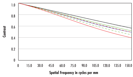
22-838 f/4 WD ∞ MTF
