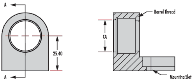
L-Slot Type (#36-410 & #36-416)
