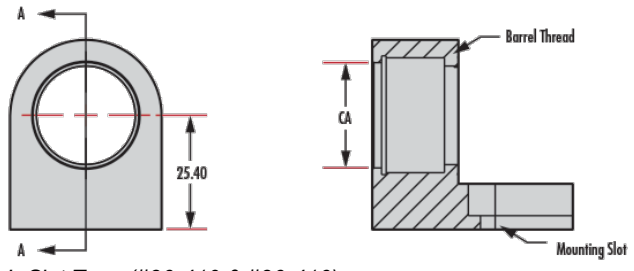
L-Slot Type (#36-410 & #36-416)
