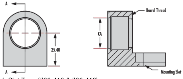
L-Slot Type (#36-410 & #36-416)
