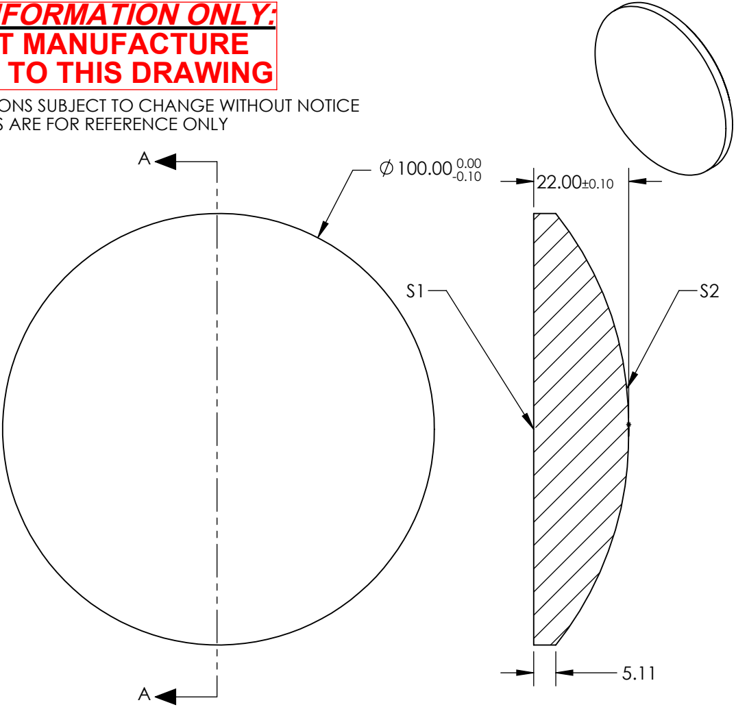
SECTION A-A
